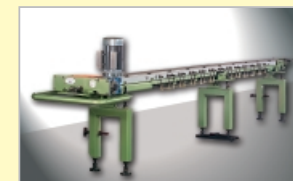
Kühlöfen-Querband für die Glasindustrie
