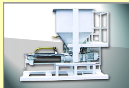
Vorbefeuchtungsstation
