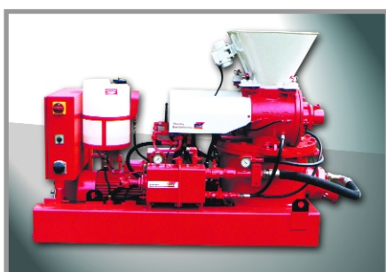
Betonspritzmaschine Typ C1N
